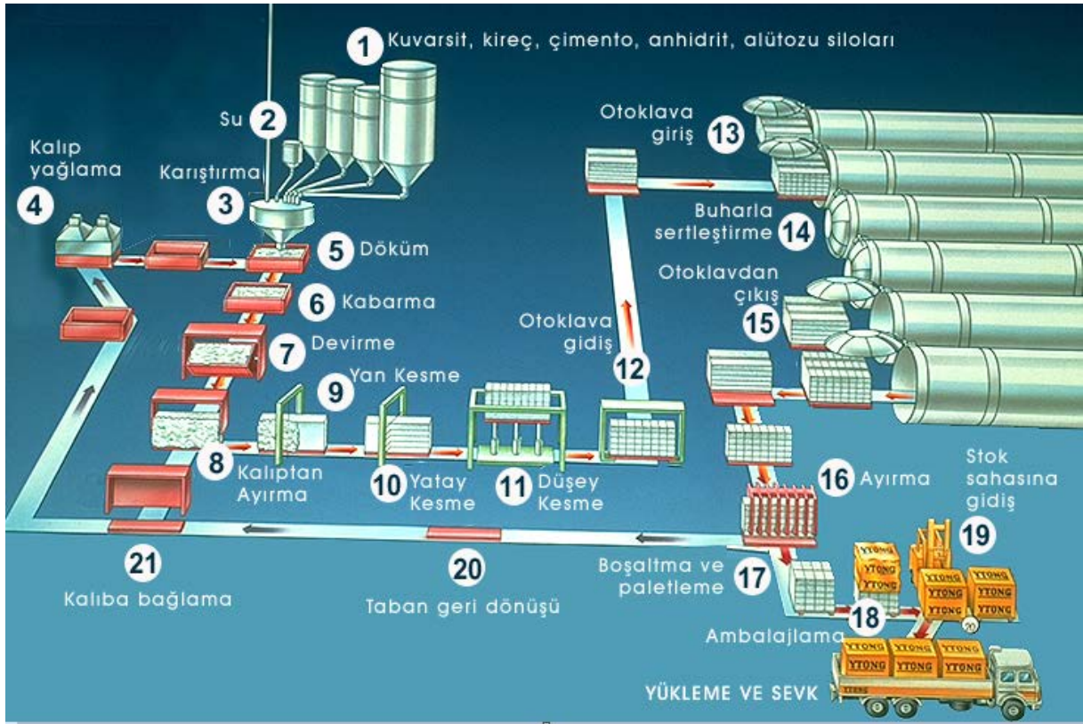
Şekil 1: Ytong Gazbeton Blok Üretimi Akış Şeması
